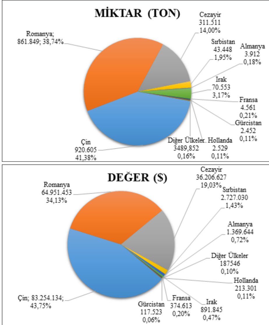
Şekil 13- Demir cevherleri ihracatında ülkelerin durumu.
