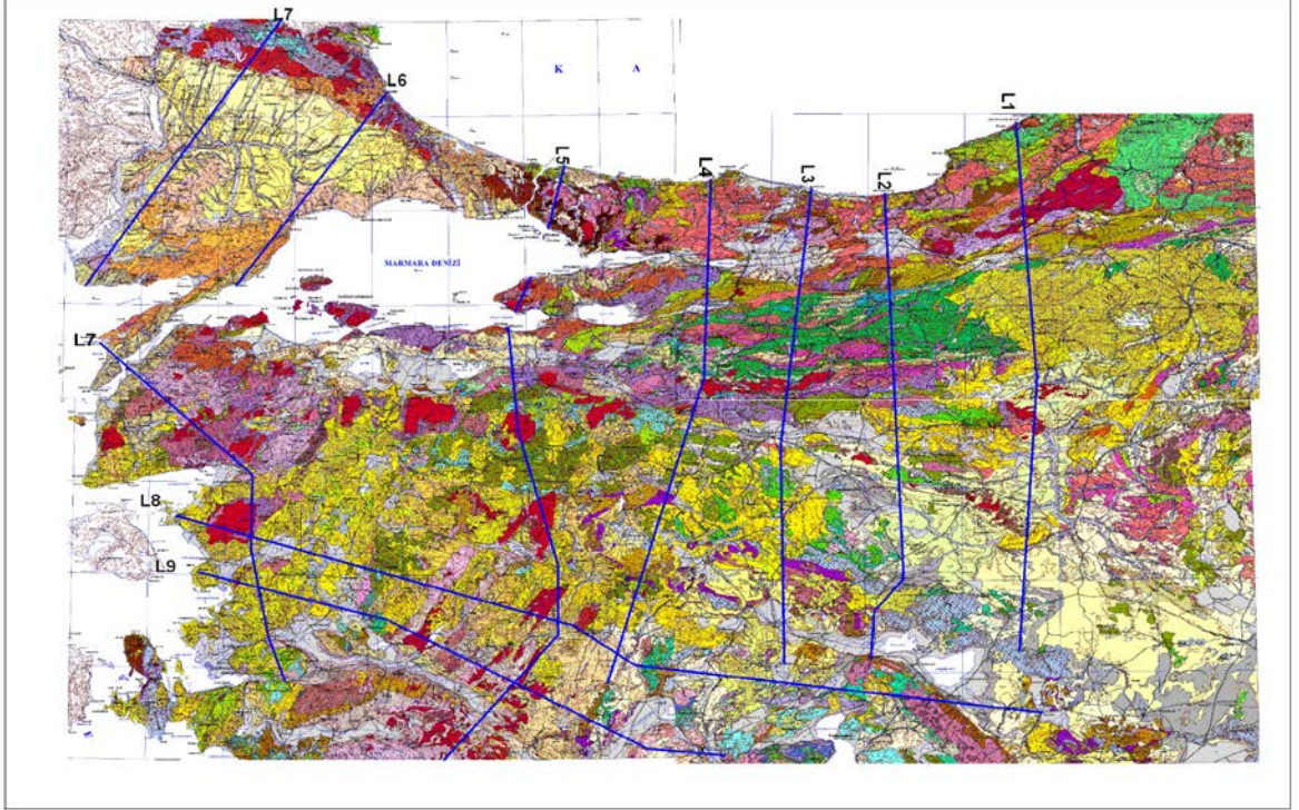
Şekil-1. Kuzey Batı Anadolu’nun Kabuk Yapısının Jeofizik Yöntemlerle Araştırılması Projesinin Gravite-Manyetotellürik ortak profilleri yer buldu haritası
