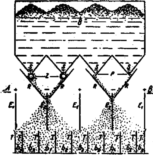
Şekil 8. Elektrostatik ayıklama tesisatı şeması.
